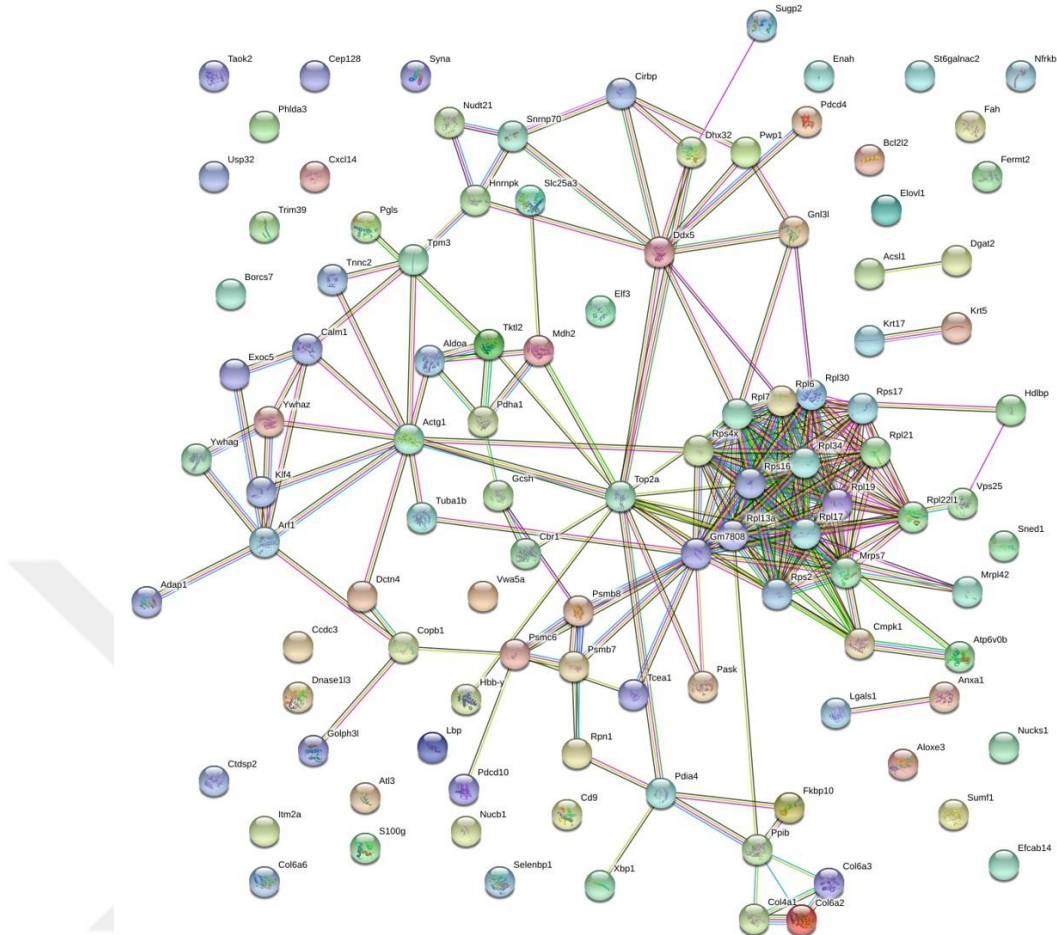
Şekil 6.4.2 STRING veri tabanı ile tanımlanan 1.gün RNA örneklerinin 0.gün RNA örneklerine göre düşük seviyede ifade edilenlerin analizi.
