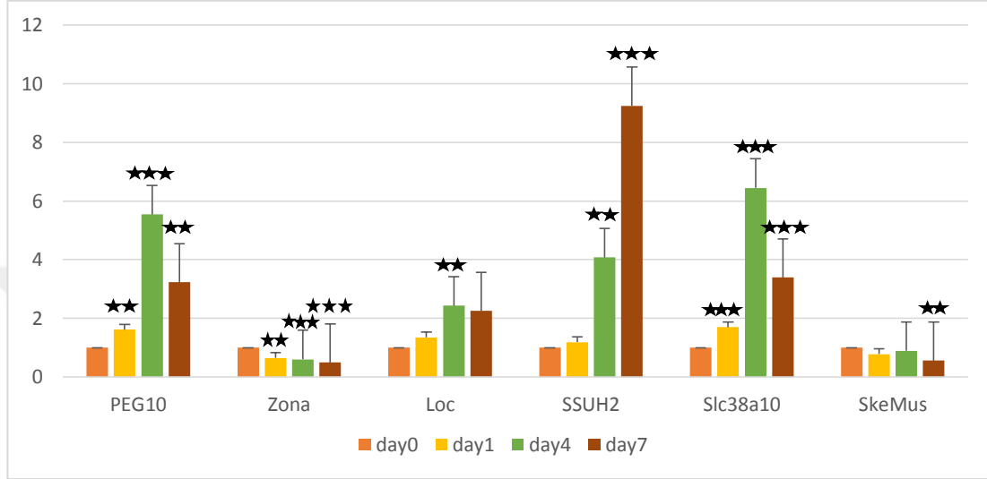
Şekil 6.2.1 Tüm zaman dilimleri için ortak olan genlerin qPCR analizi.
