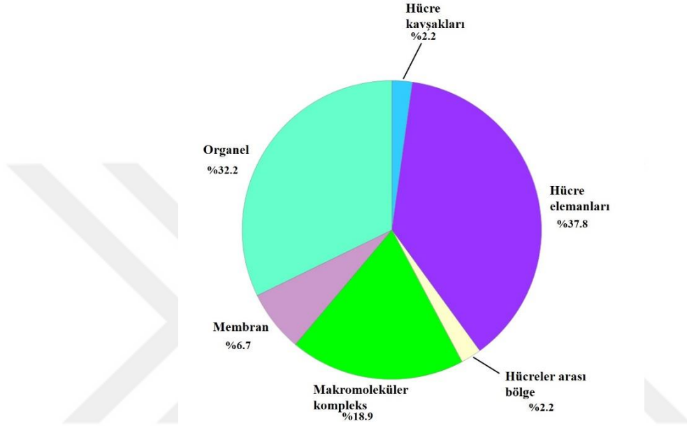
Şekil 8.7 PANTHER veri tabanı ile tanımlanan 7.gün RNA örneklerinin 0.gün RNA örneklerine göre hücresel bileşen analizi.
