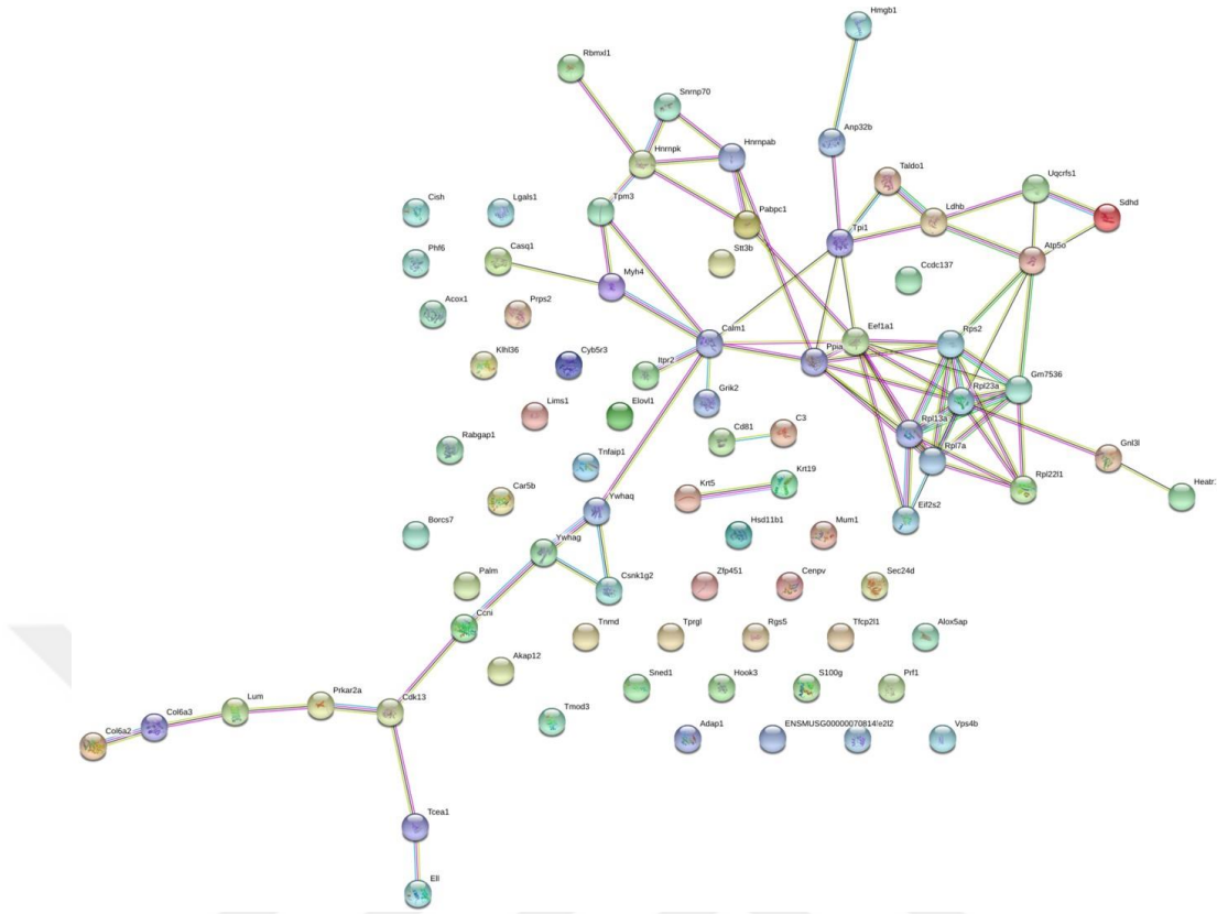
Şekil 6.4.4 STRING veri tabanı ile tanımlanan 4.gün RNA örneklerinin 0.gün RNA örneklerine göre düşük seviyede ifade edilenlerin analizi.
