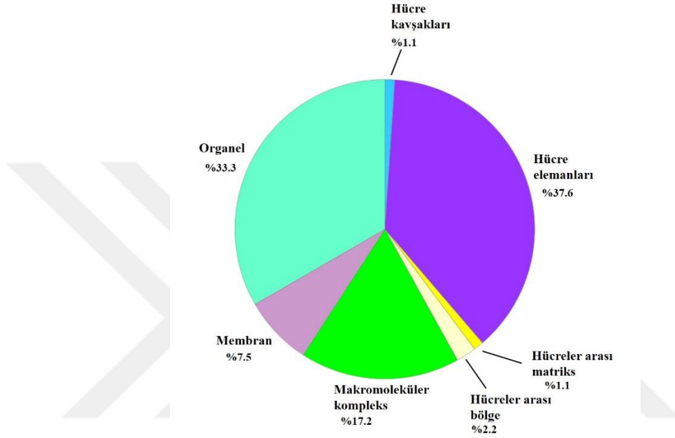
Şekil 8.1 PANTHER veri tabanı ile tanımlanan 1.gün RNA örneklerinin 0.gün RNA örneklerine göre hücresel bileşen analizi.
