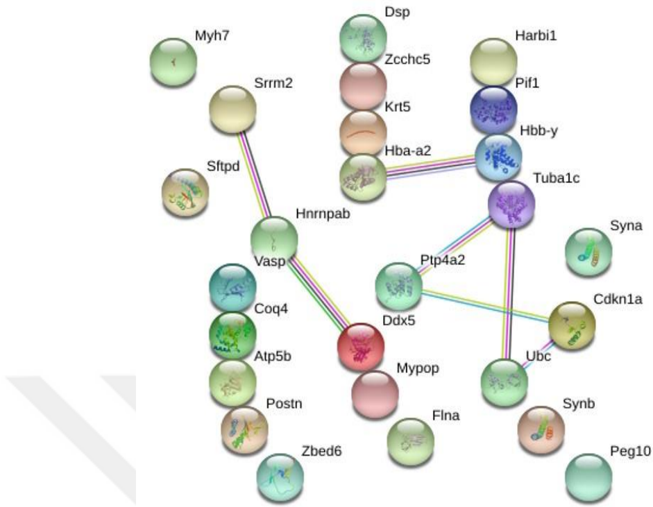
Şekil 6.4.1 STRING veri tabanı ile tanımlanan 1.gün RNA örneklerinin 0.gün RNA örneklerine göre yüksek seviyede ifade edilenlerin analizi.
